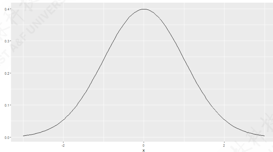
理论正态分布图
