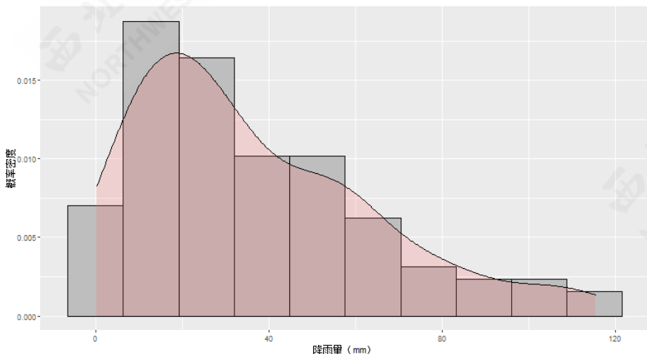
降雨量记录数据的分布图 n=100
